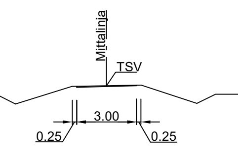
J2 Peruspoikkileikkaus 1:200 PLV 1805-1996
