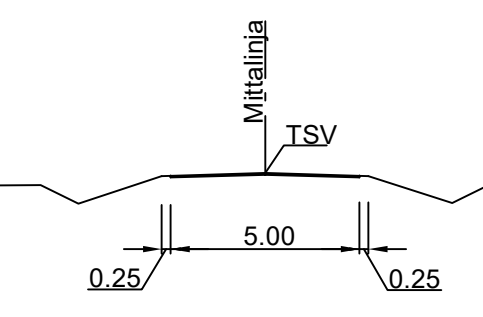
M6 Peruspoikkileikkaus 1:200 PLV 1500-1805
