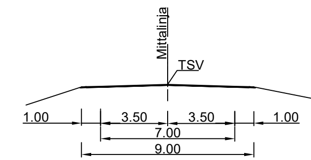
M6 Peruspoikkileikkaus 1:200 PLV 0-1500
