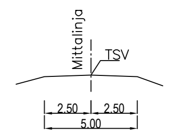
Y23 PERUSPOIKKILEIKKAUS 1:200
