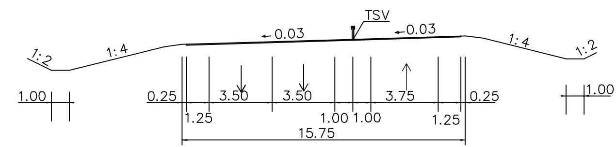
V8 PERUSPOIKKILEIKKAUS 1:200
