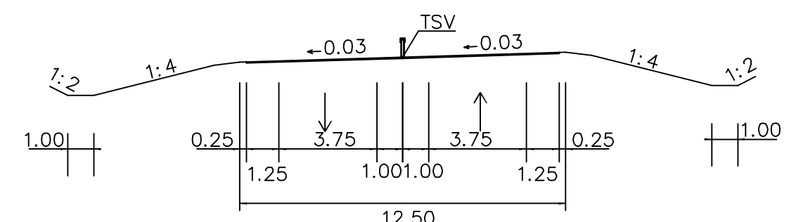
V8 PERUSPOIKKILEIKKAUS 1:200
