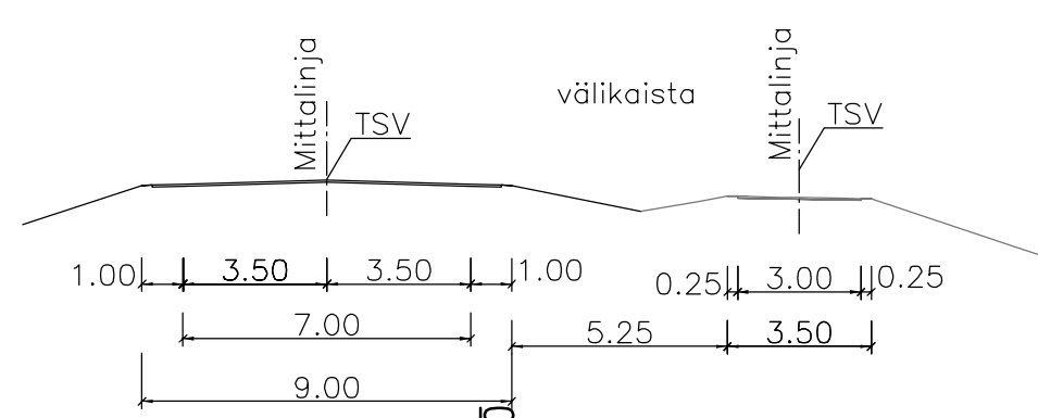
M2 JA J1 PERUSPOIKKILEIKKAUS 1:200
