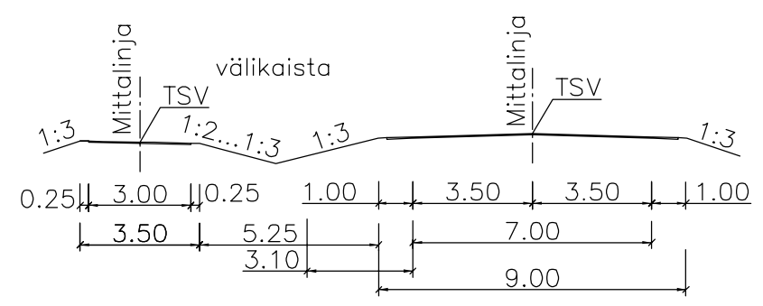
M1 JA J1 PERUSPOIKKILEIKKAUS 1:200
