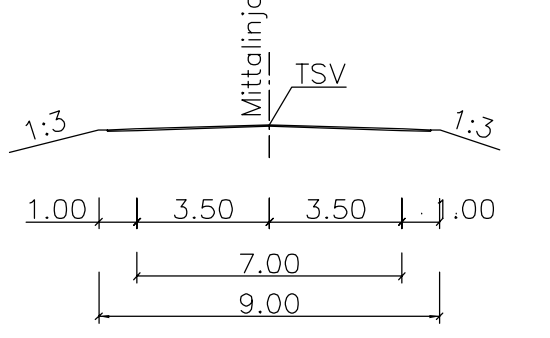
M1 PERUSPOIKKILEIKKAUS 1:200
